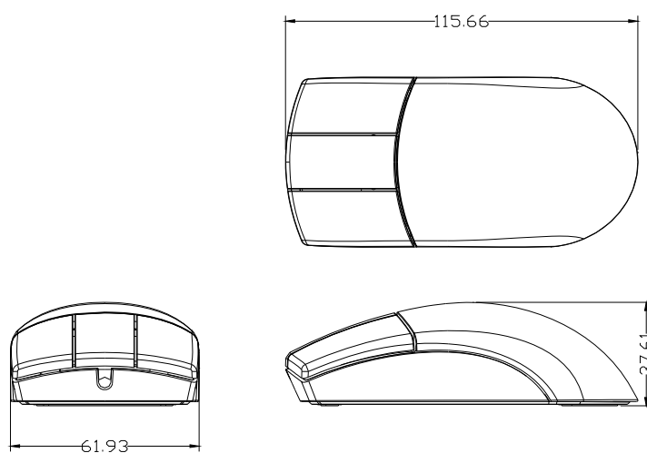
3ボタンマウス[N8052-FS06]、[N8052-01]
