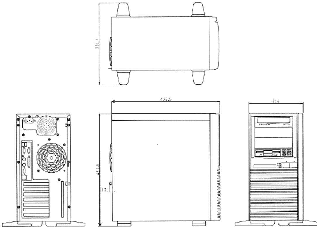
外形寸法：216(W)×433(D)×452(H) mm (スリッパは含まず)
