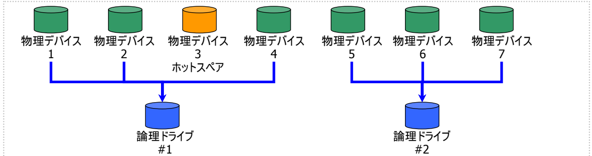
図 16 [イージーコンフィグレーション] 物理デバイスの割り当て 1
